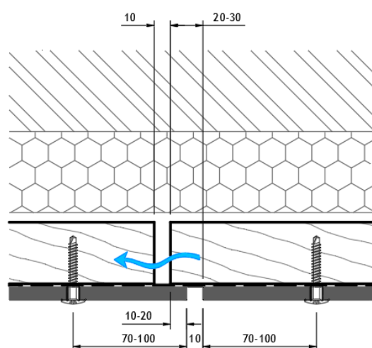
Coupe horizontale du plafond
