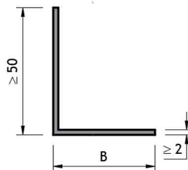
Tussenprofiel
